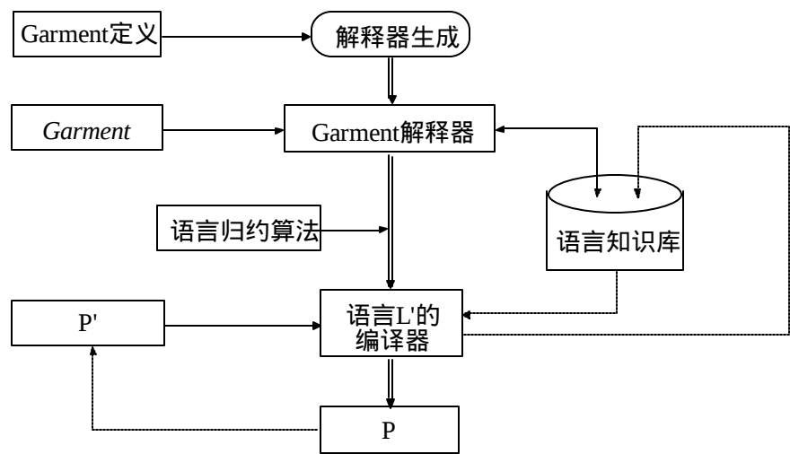
图2. Garden的工作流程
