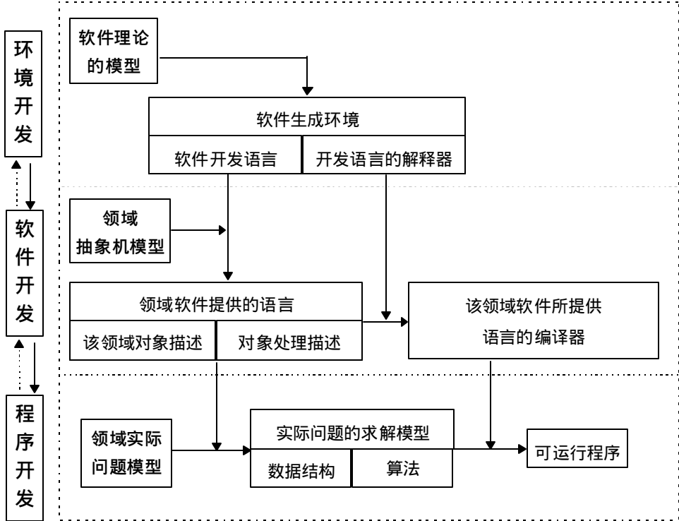
图 1. 环境开发、软件开发和程序开发
