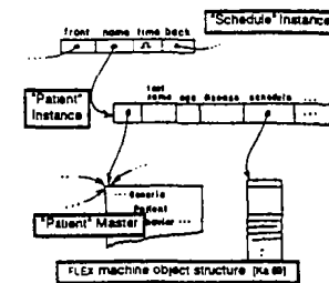
FLEX machine object structure (Ka 69)
